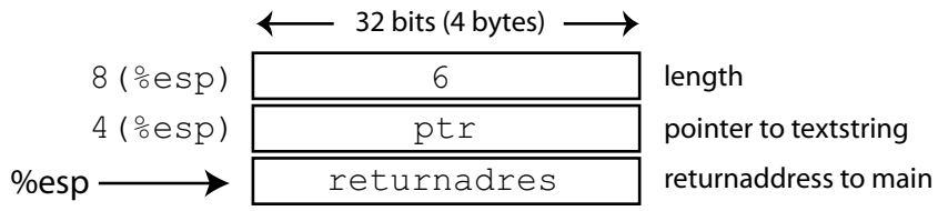
Figuur 23.2 Twee parameters in het stackframe
