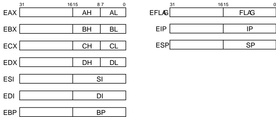
Figuur 23.1 Registerset van de 386
