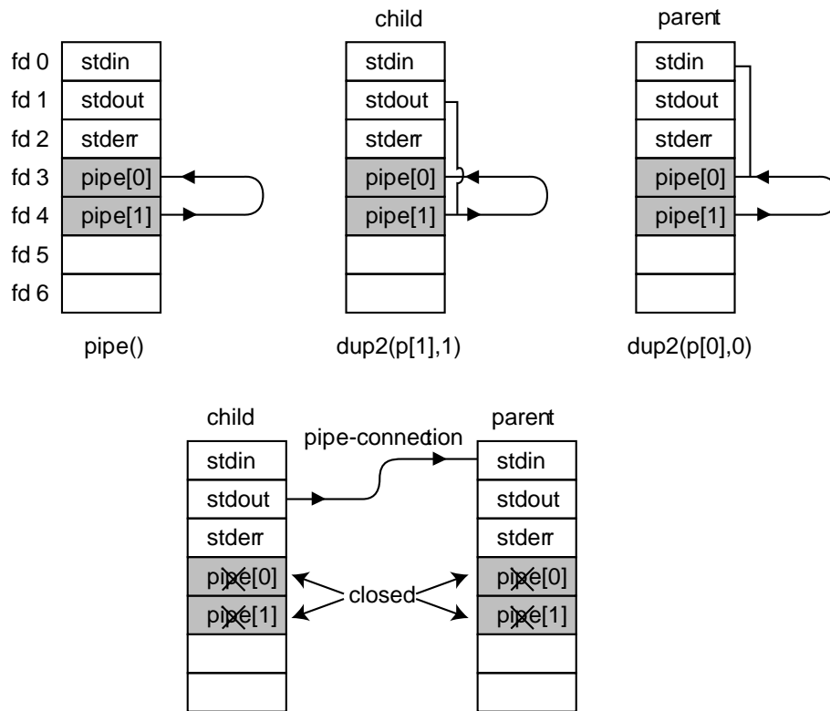
Figuur 22.3 Omleiding van stdin en stdout via pipe en dup2
