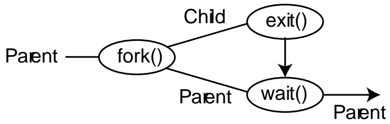
Figuur 22.2 De systeemaanroep fork in combinatie met wait
