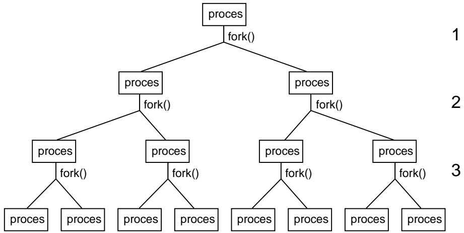
Figuur 22.1 Het effect van drie fork-systeemaanroepen op rij
