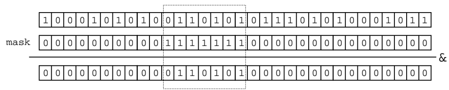
Figuur 12.3 Selectie van zeven bits met een bitmasker
