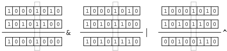
Figuur 12.1 De bitgewijze bewerkingen AND, OR en EXOR
