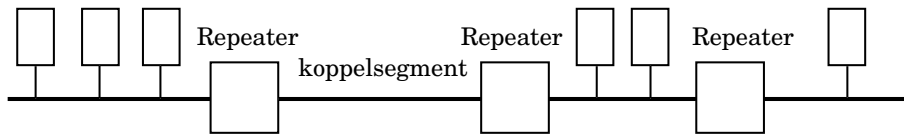
Figuur 16.8 Segmenten en repeaters van de Profibus
