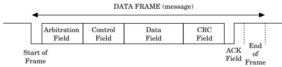
Figuur 16.5 Opbouw van een CAN frame
