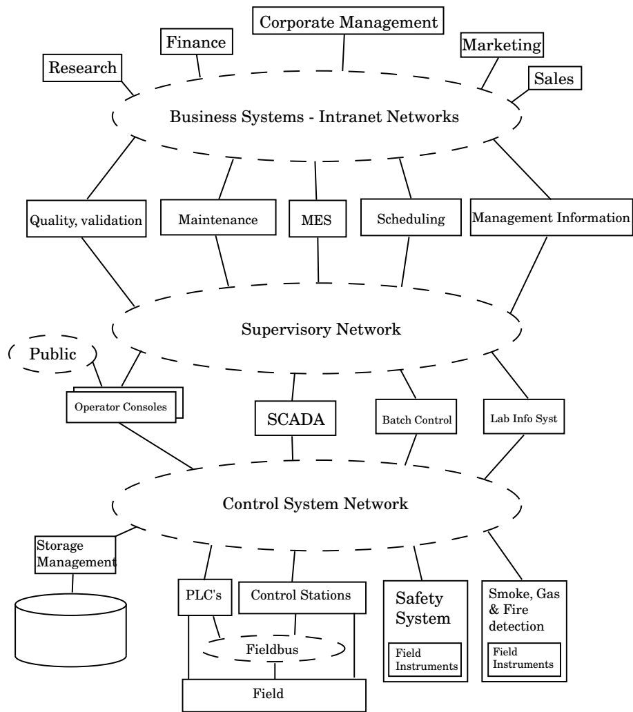
Figuur 16.2 Uitgewerkt model van een productie omgeving Computersystemen en embedded systemen (LvM)
