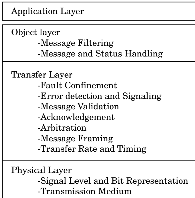
Figuur 16.4 Lagenstructuur van CAN
