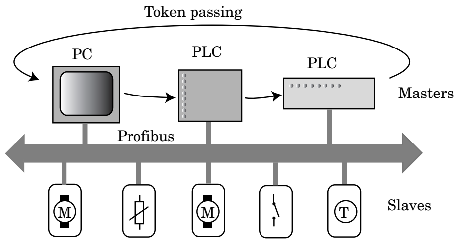
Figuur 16.7 Configuratie op basis van Profibus
