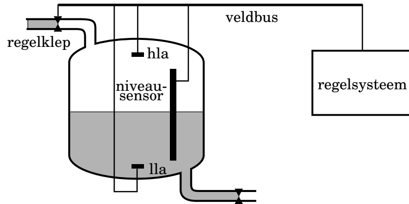
Figuur 16.3 Niveauregelaar met een veldbus Computersystemen en embedded systemen (LvM)
